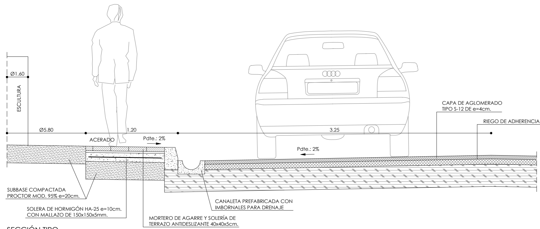
SECCIÓN TIPO ESCALA: 1/25
